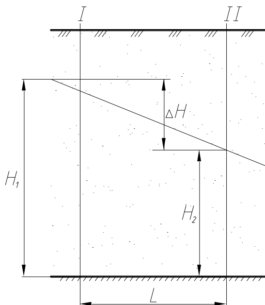
Рис.1. Схема движения (фильтрации) грунтовой воды.
