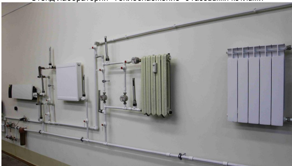
Стенд "Система отопления" с различными отопительными приборами
