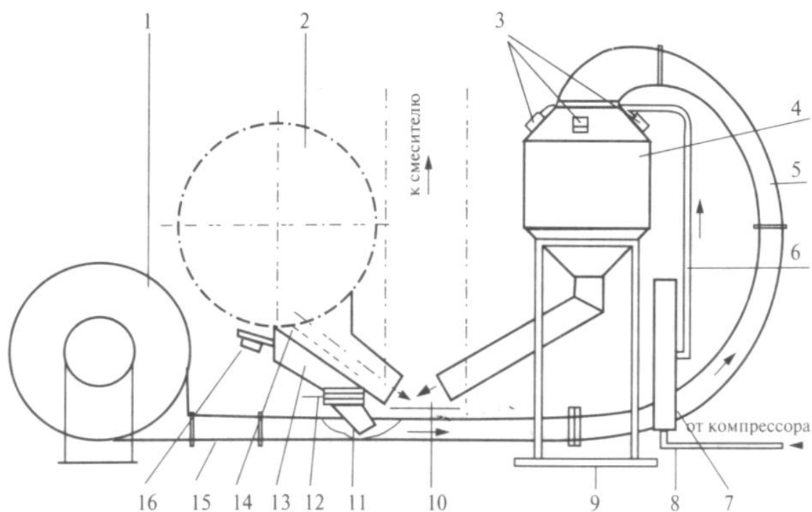
Рисунок 6.4 – Опытно-промышленная установка для трибоактивации песков: – вентилятор высокого давления, 2 – сушильный барабан, 3 – форсунки для ПАВ, 4 – циклон, 5 – трубопровод-активатор, 6 – трубопровод для ПАВ, 7 – бак для ПАВ, 8 – трубопровод для сжатого воздуха, 9 – стойка, 10 – горячий элеватор, 11 – диффузор, 12 – задвижка, 13 – бункер, 14 – сетка, 15 – переходник, 16 – вибратор
