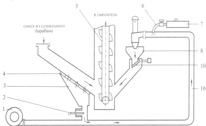
Рисунок 6.3 – Технологическая линия для получения трибоактивированных песков: 1 – вентилятор, 2 – шиберная задвижка, 3 – приемный бункер песка, 4 – вибрирующая металлическая сетка, 5 – горячий элеватор, 6 – устройство для подачи ПАВ, 7 – емкость для ПАВ, 8 – циклон, 9 – дроссельная заслонка, 10 – трубопровод-активатор
