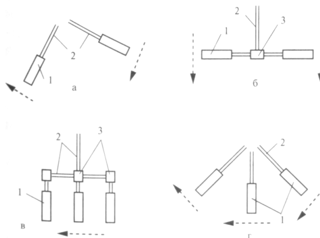
Рисунок 9.3 – Схема размещения смесительных установок: а – раздельная, б – прямолинейная, в – параллельная, г - кольцевая; 1 – смеситель; 2 – транспортер; 3 – накопительный бункер (стрелками указано направление движения автомобилей-самосвалов)
