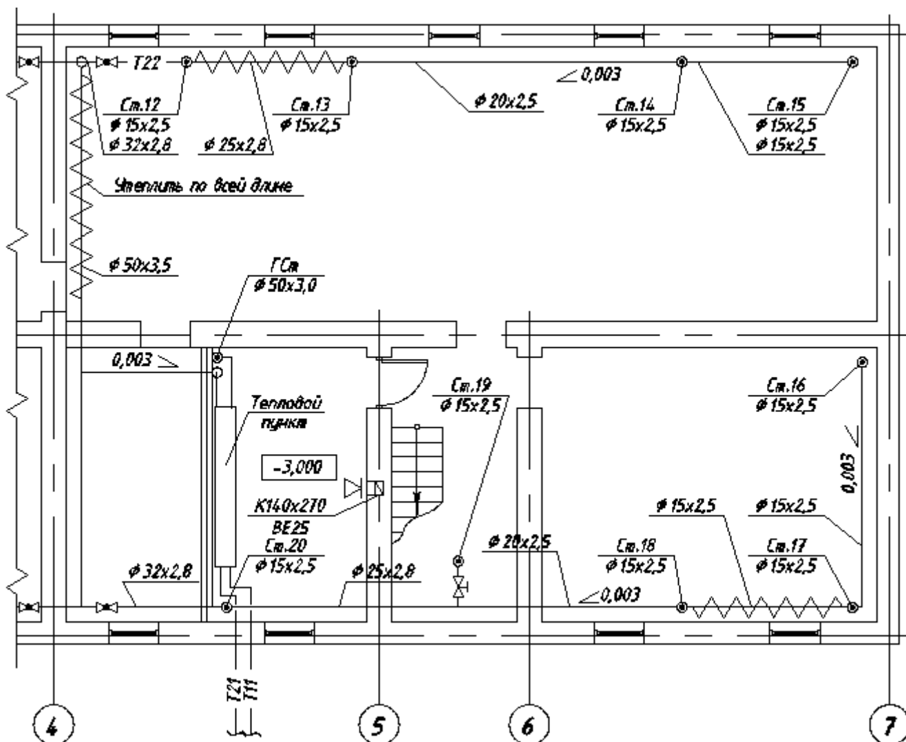
Рис. 8 Пример расположения элементов системы отопления и вентиляции на плане подвала
