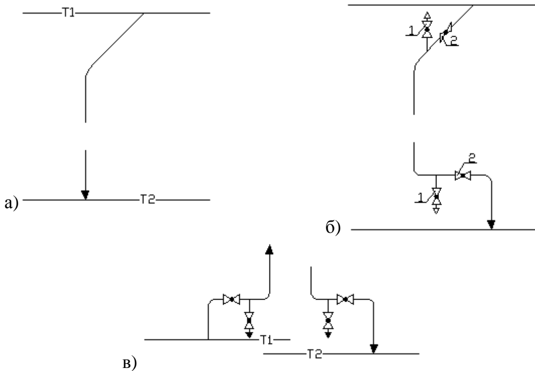
Рис. 5 Схемы присоединения стояков к магистралям зданий различной этажности: а – двух-трехэтажных, б – четырех-семиэтажных с верхней разводкой, в – с нижней разводкой. 1 – спускной кран, 2 – запорный кран.
