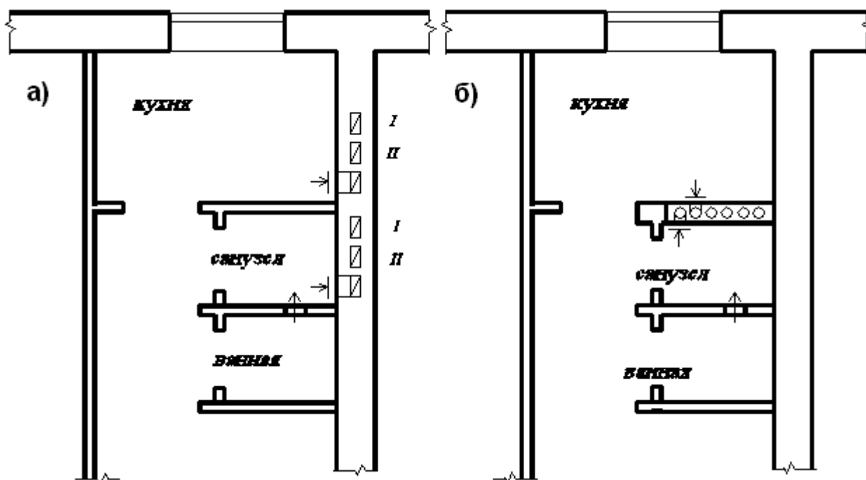
Рис. 15. Устройство вентиляционных каналов: а) во внутренних кирпичных стенах; б) с использованием вентиляционных панелей
