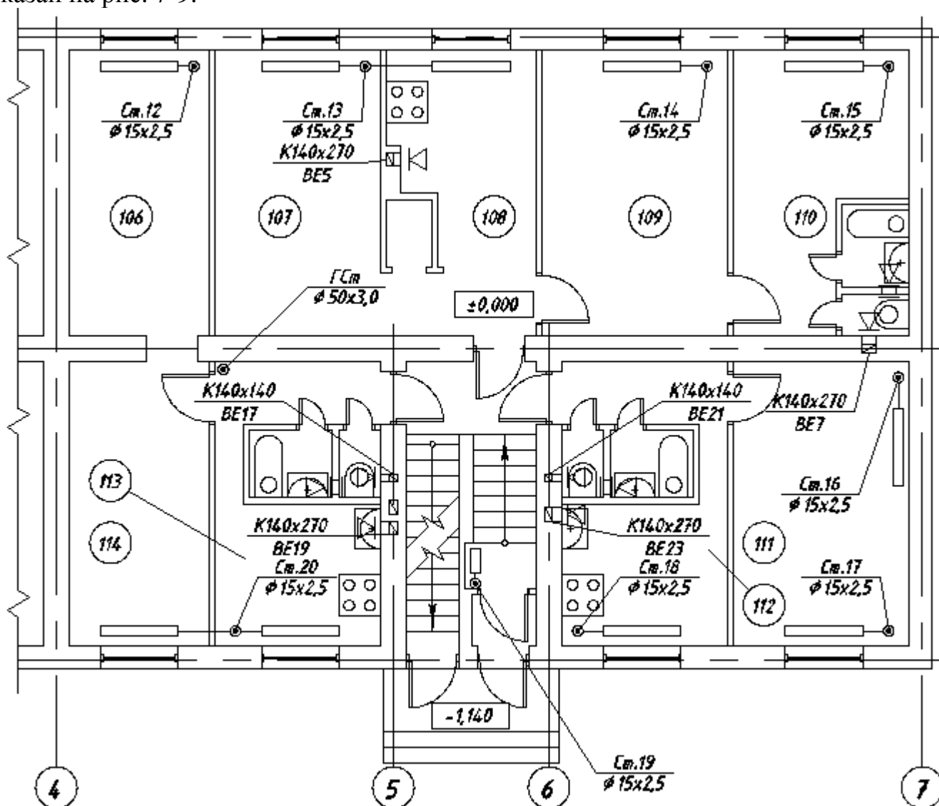
Рис. 7 Пример расположения элементов системы отопления и вентиляции на плане этажа
