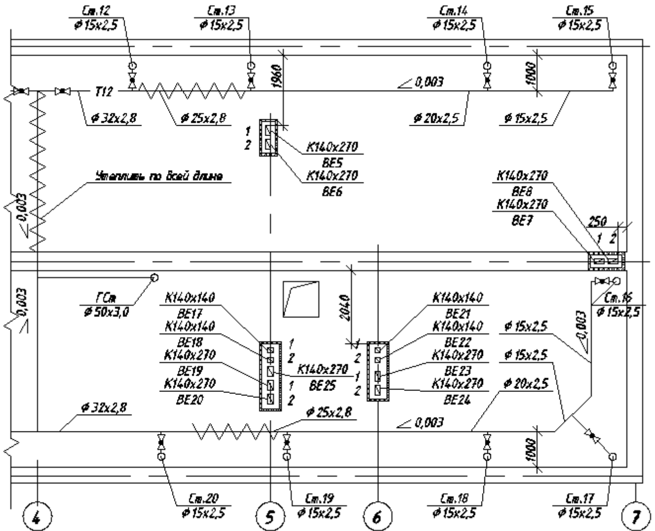
Рис. 9 Пример расположения элементов системы отопления и вентиляции на плане чердака
