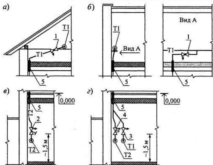
Рис. 6 Некоторые элементы конструкции систем отопления а)- подсоединение стояка к подающей магистрали на чердаке с двухскатной кровлей, б)-то же с плоской кровлей, в)- подсоединение стояка к обратной магистрали в подвале, г)- подсоединение стояков при нижней разводке 1-кран шаровой, 2-клапан балансировочный, 3-кран шаровой для слива воды из стояка, 4-клапан балансировочный (или регулятор перепада давления для двухтрубной системы), 5-гильза.
