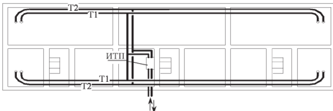
Рис. 4 Расположение магистралей тупиковой системы отопления с нижней разводкой в зданиях шириной более 9 метров
