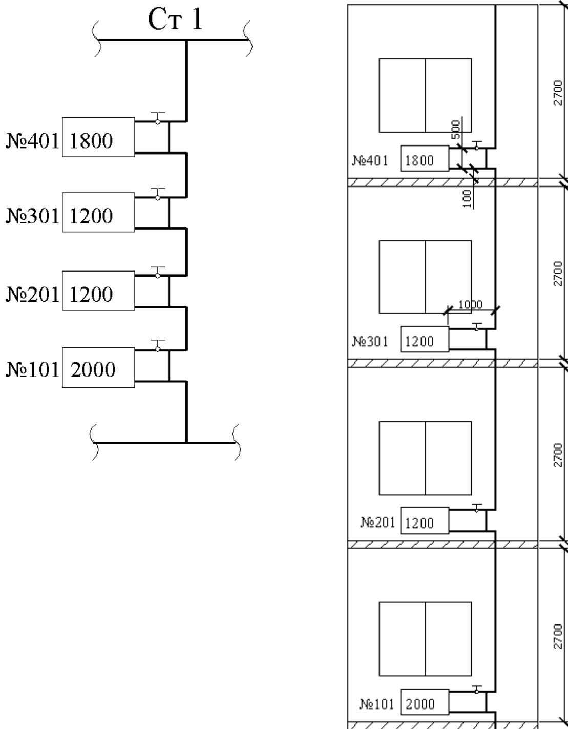
Рис. 15 Схема стояка к примеру 5
