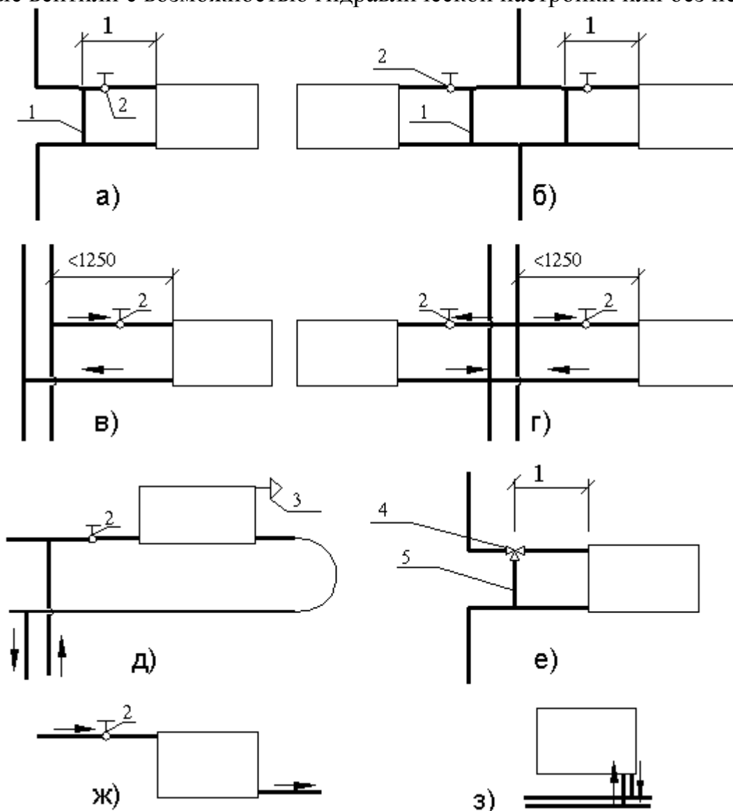
Рис. 10 Присоединение отопительных приборов к стоякам вертикальных систем отопления: а) и б) - однотрубных, в) и г) - двухтрубных, д) - к верхним приборам стояков с нижней разводкой магистралей двухтрубной системы, е) - однотрубных проточно-регулируемых, ж) – разносторонне присоединение при большой длине прибора, з) – нижнее присоединение (для приборов со встроенным терморегулятором).
