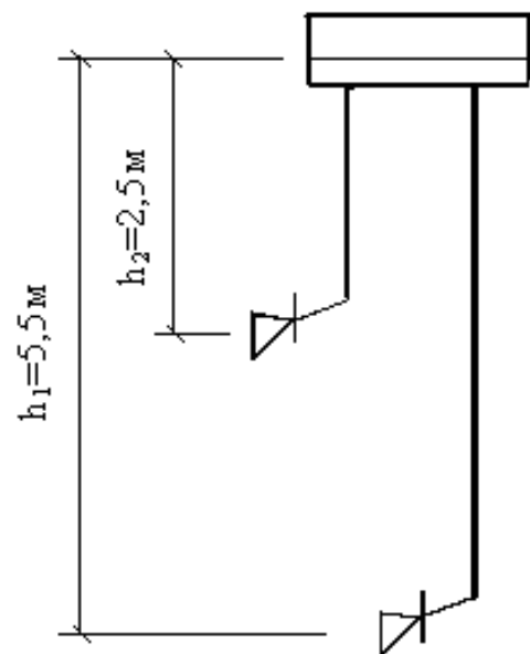
Рис. 16. Схема системы вентиляции
