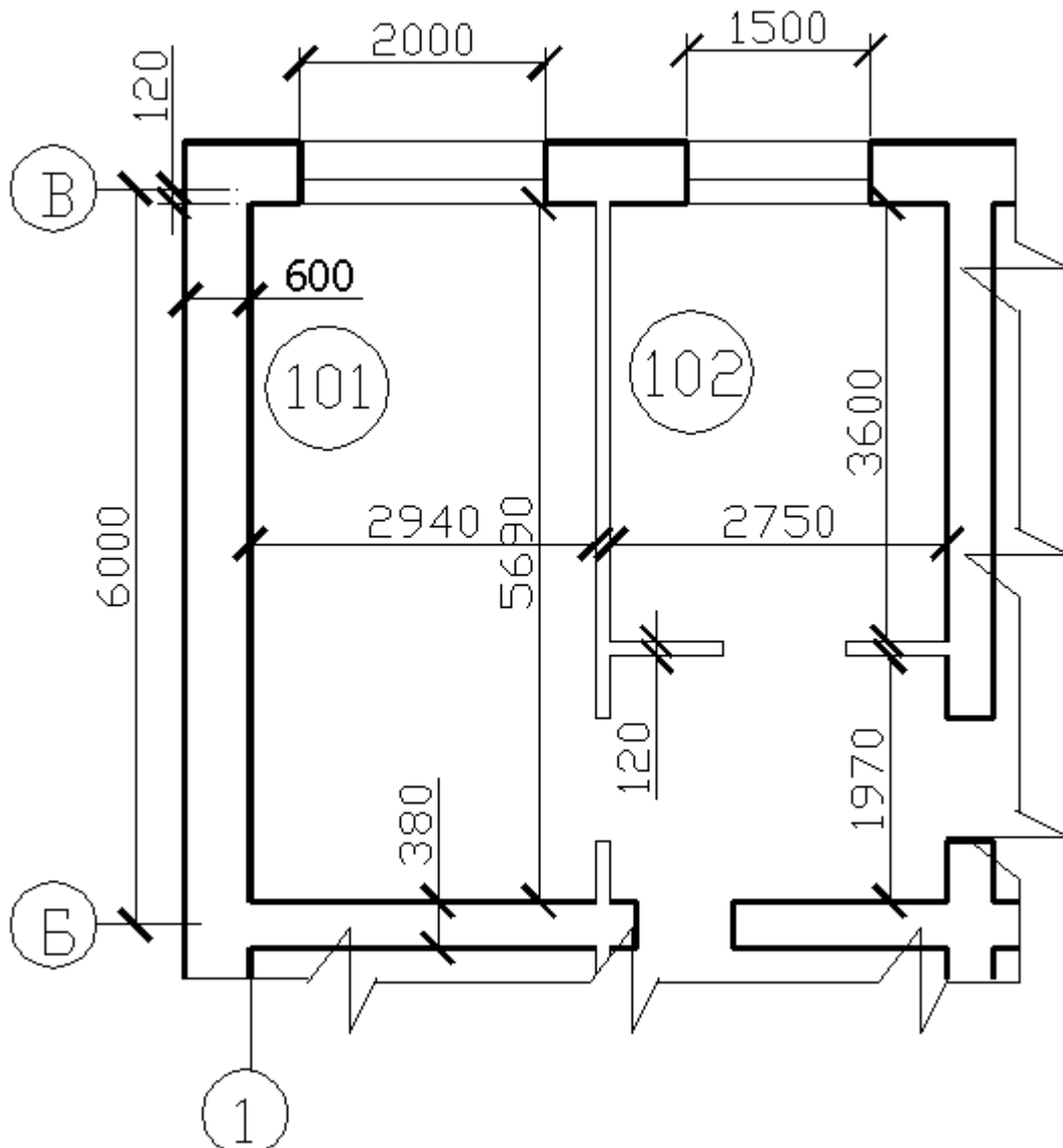
Рис. 2 План части здания к примеру 1
