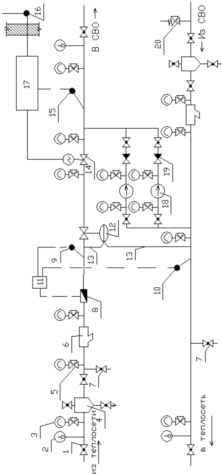
Рис. 13 Схема ИТП со смесительным насосом, включенным в перемычку. 1–шаровой кран, 2–термометр, 3–манометр, 4–грязевик, 5–трехходовой кран, 6–фильтр, 7–контрольно-спускной кран, теплосчетчик : 8–счетчик воды, 9–датчик температуры горячей воды, 10–датчик температуры охлажденной воды, 11–вычислительный блок; 12–регулятор перепада давления, 13–импульсная трубка, регулятор теплового потока : 14–двухходовой клапан с электроприводом, 15–датчик температуры горячей воды, 16– датчик температуры наружного воздуха, 17–блок автоматизации; 18–смесительный насос, 19–обратный клапан, 20–предохранительный клапан.
