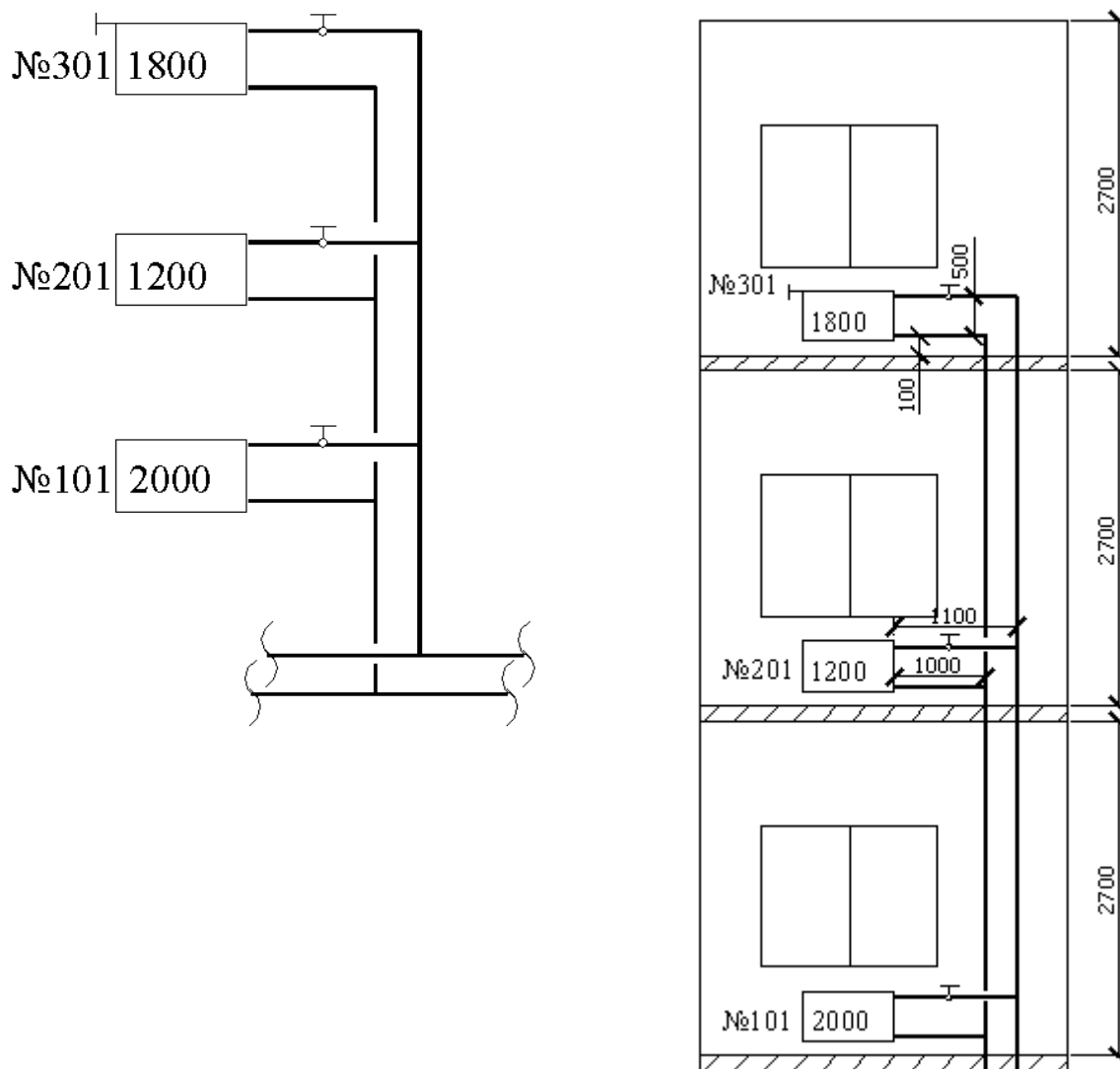
Рис. 14 Схема стояка к примеру 4
