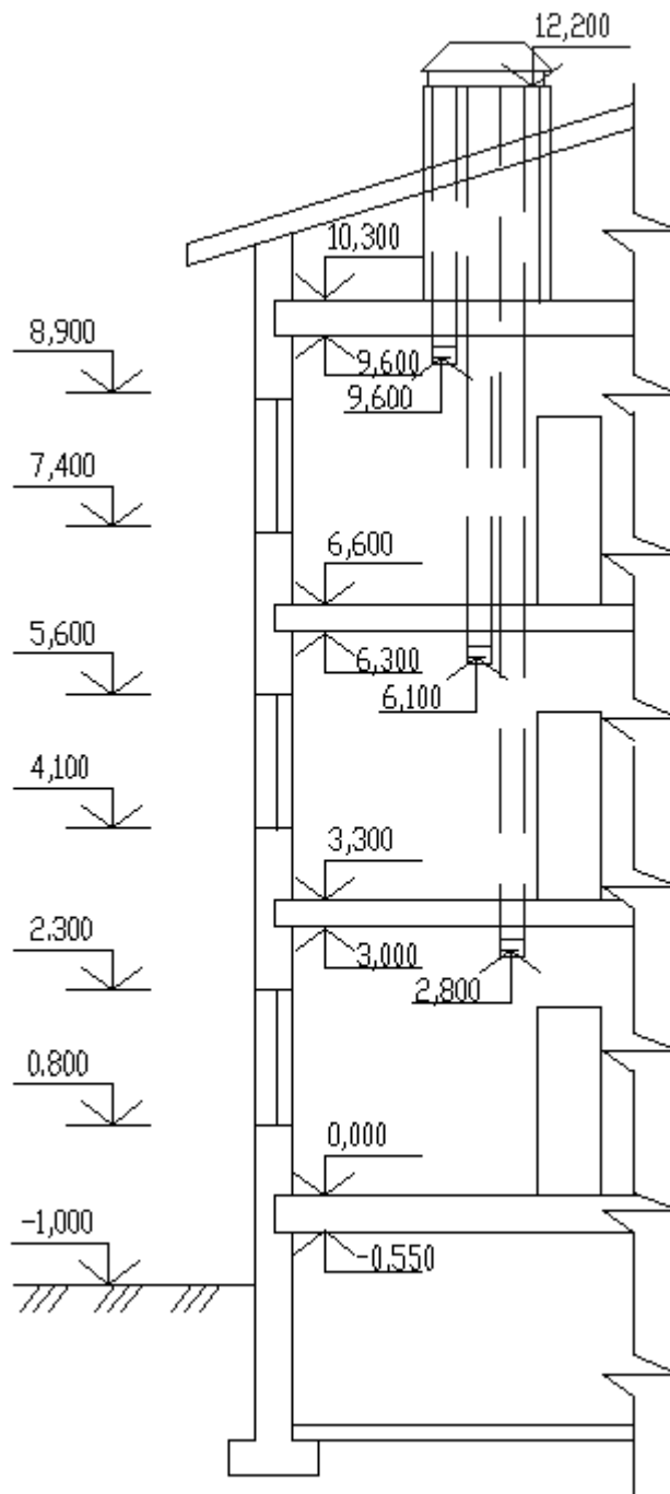
Рис. 3 Разрез здания к примеру 1
