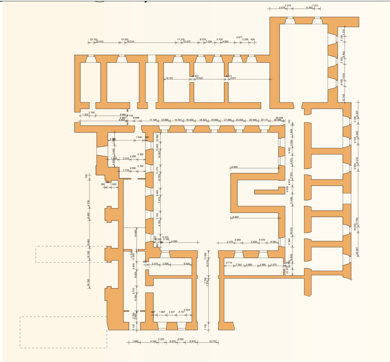
Рис. 1. Обмерные чертежи
